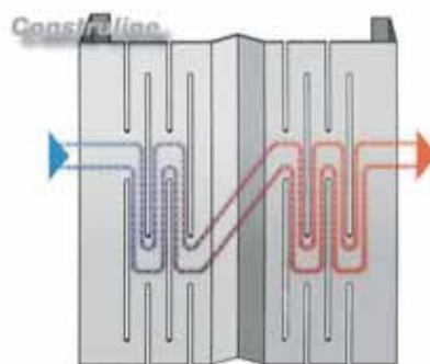
Typická skladba stěny šířky 245 mm
