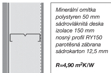
Typická skladba stěny šířky 245 mm
